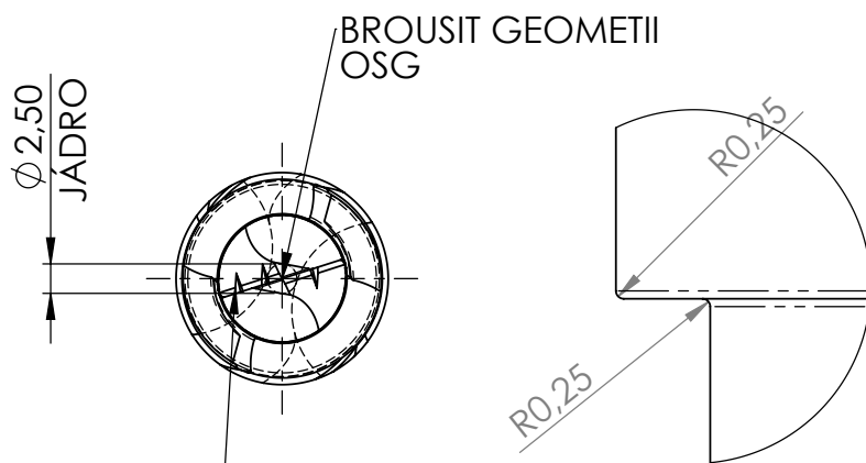
DETAIL J MĚŘÍTKO 4 : 1
